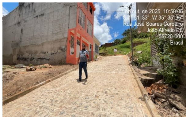
FOTO 16: Pavimentação na Rua Maria Auzira 01.
