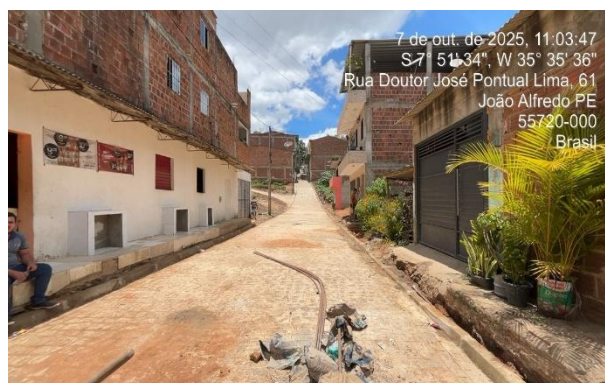
FOTO 28: Pavimentação na Rua Maria Feliciano da Silva.
